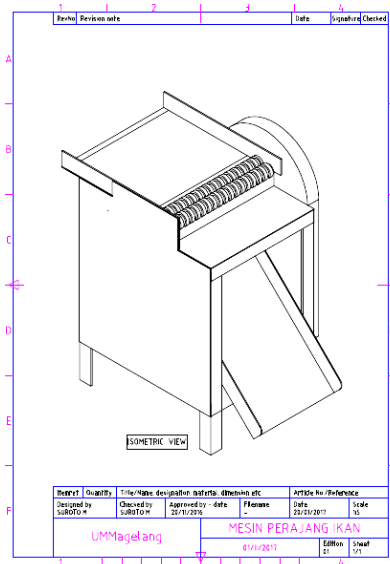
Gambar 2. Rancangan Mesin.
