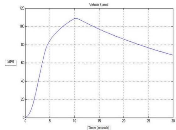
Gambar 12. Hasil simulasi vehicle speed saat perlambatan dimulai pada kecepatan 110 mph
