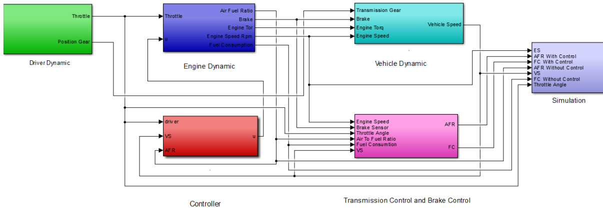
Gambar 6 . Pemodelan AFR dengan kontrol mesin dan transmisi.
